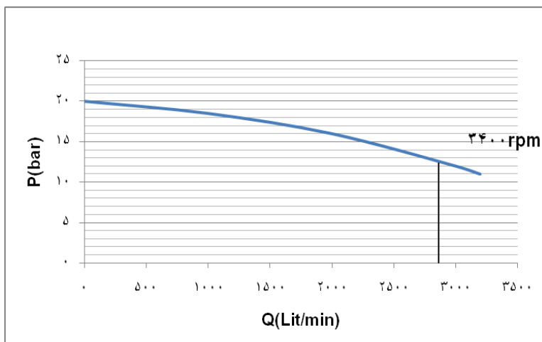
نمودار عملکرد پمپ ۳۰۰۰
